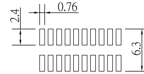
P.C.Board Layout
