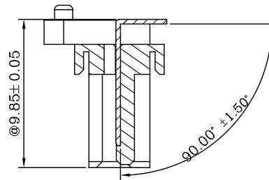
端子折彎後半成品視圖
